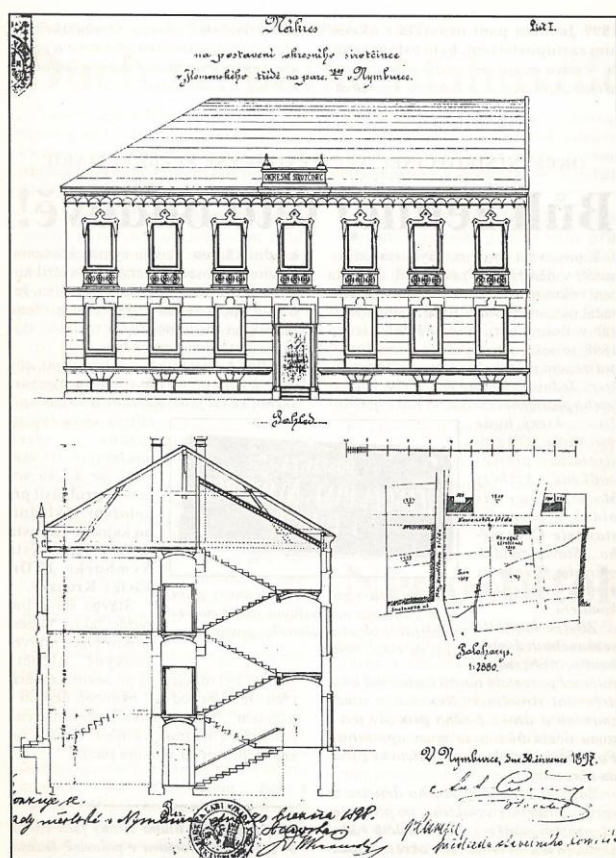
Výkres s pohledem, řezem a polohorysem potvrzený městskou radou a stavebním komitétem.
